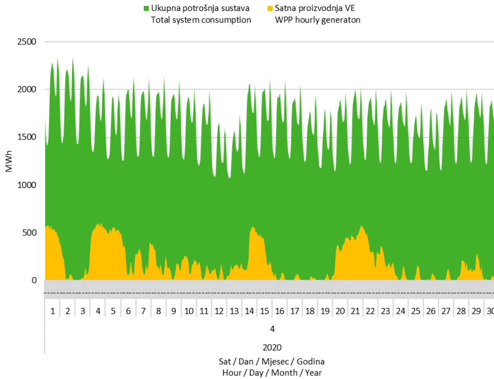
Slika 7 Usporedba satnog dijagrama opterećenja sustava i proizvodnje vjetroelektrana u travnju 2020. godine
