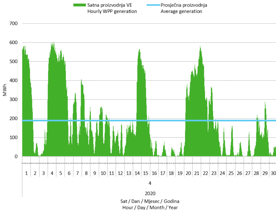
Slika 2 Satna proizvodnja svih vjetroelektrana u travnju 2020. godine
