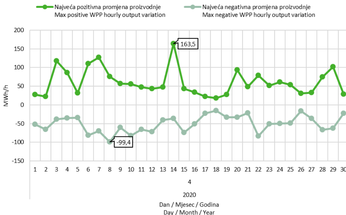
Slika 9 Maksimalna pozitivna i maksimalna negativna promjena satne proizvodnje VE u travnju 2020. godine
