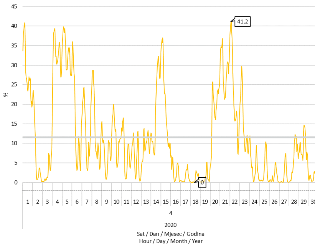
Slika 8 Udio proizvodnje vjetroelektrana u pokrivanju satnog opterećenja elektroenergetskog sustava u travnju 2020. godine
