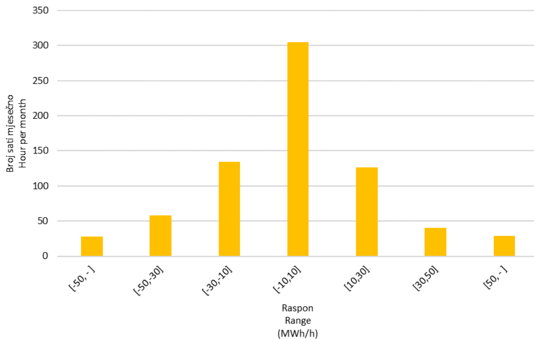
Slika 10 Statistička raspodjela satnih promjena proizvodnje VE u travnju 2020. godine
