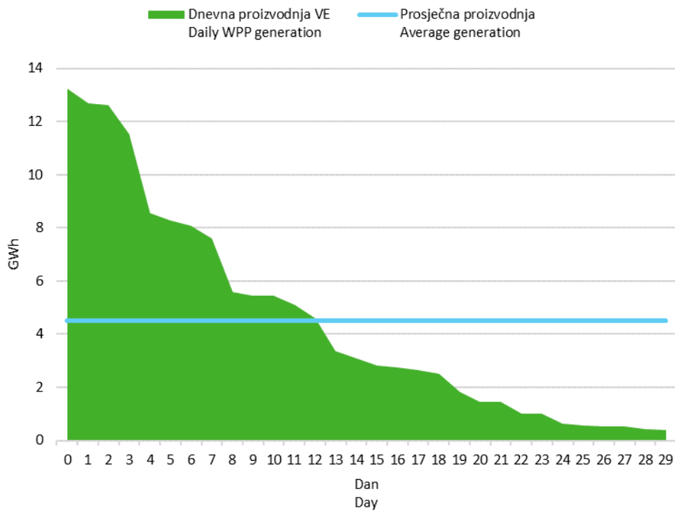
Slika 6 Krivulja trajanja dnevne proizvodnje vjetroelektrana u travnju 2020. godine
