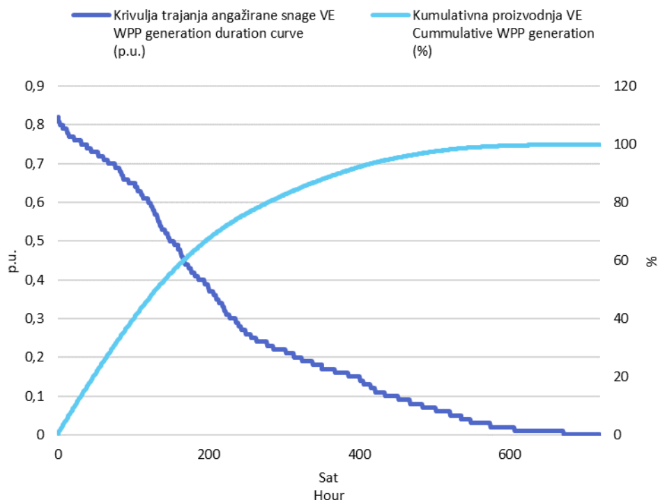
Slika 3 Krivulja trajanja angažirane snage svih VE i kumulativna proizvodnja VE u travnju 2020. godine u jediničnim vrijednostima
